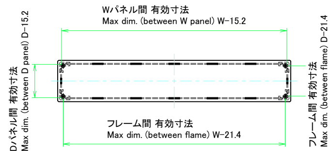
下カバー / Bottom cover
